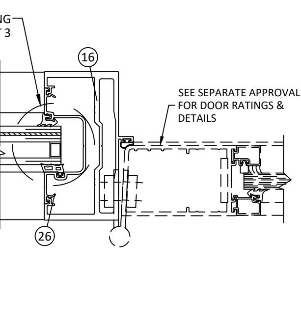
M 10 HORIZONTAL SECTION DOOR JAMB MULLION
